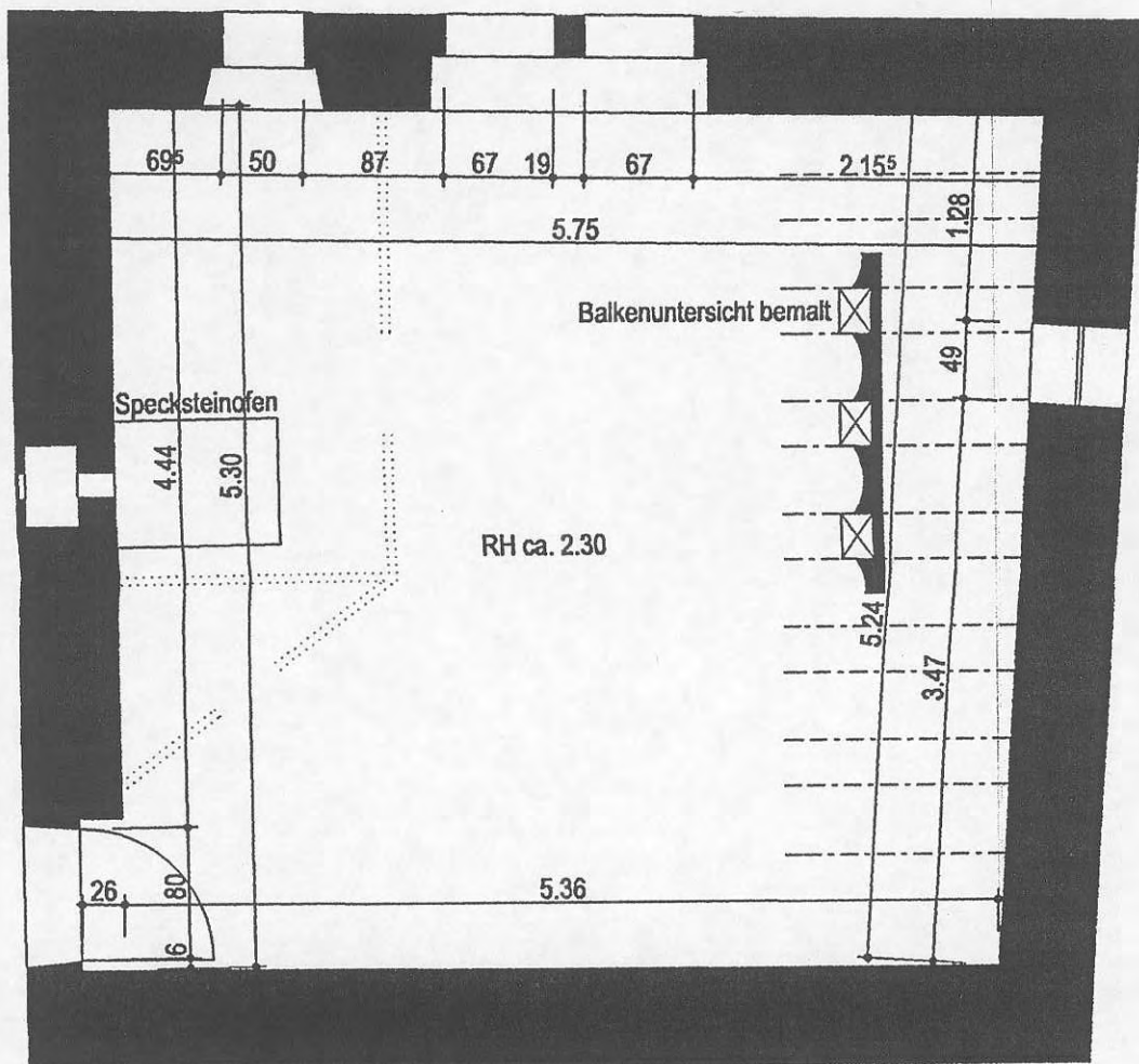
OBERGESCHOSS
