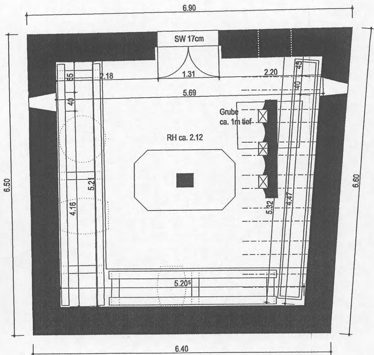
KELLERGECHOSS
