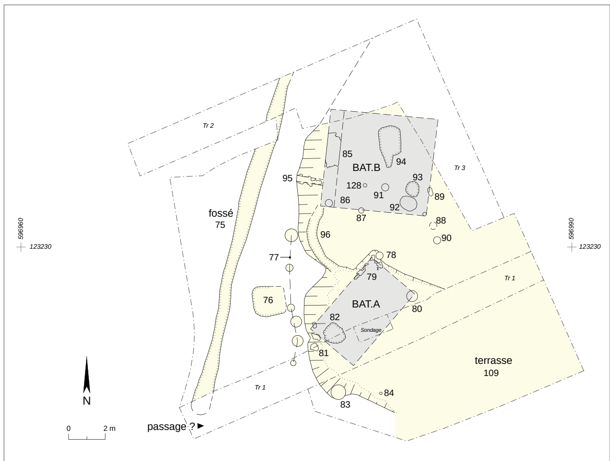
Fig. 17. AF09, maison Gandolfi. Plan des vestiges romains.
