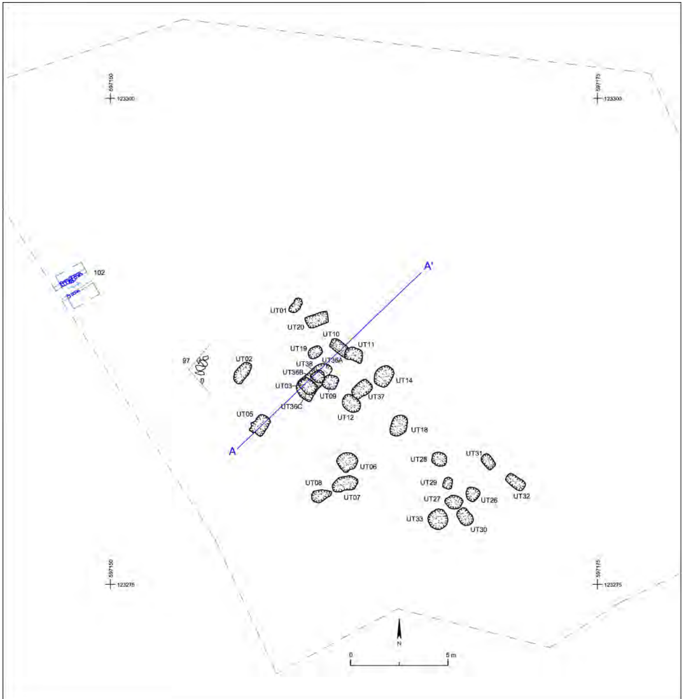
Fig. 8. AF08, maison Délitroz. Plan des vestiges et situation de la coupe schématique A-A' (fig. 9).
