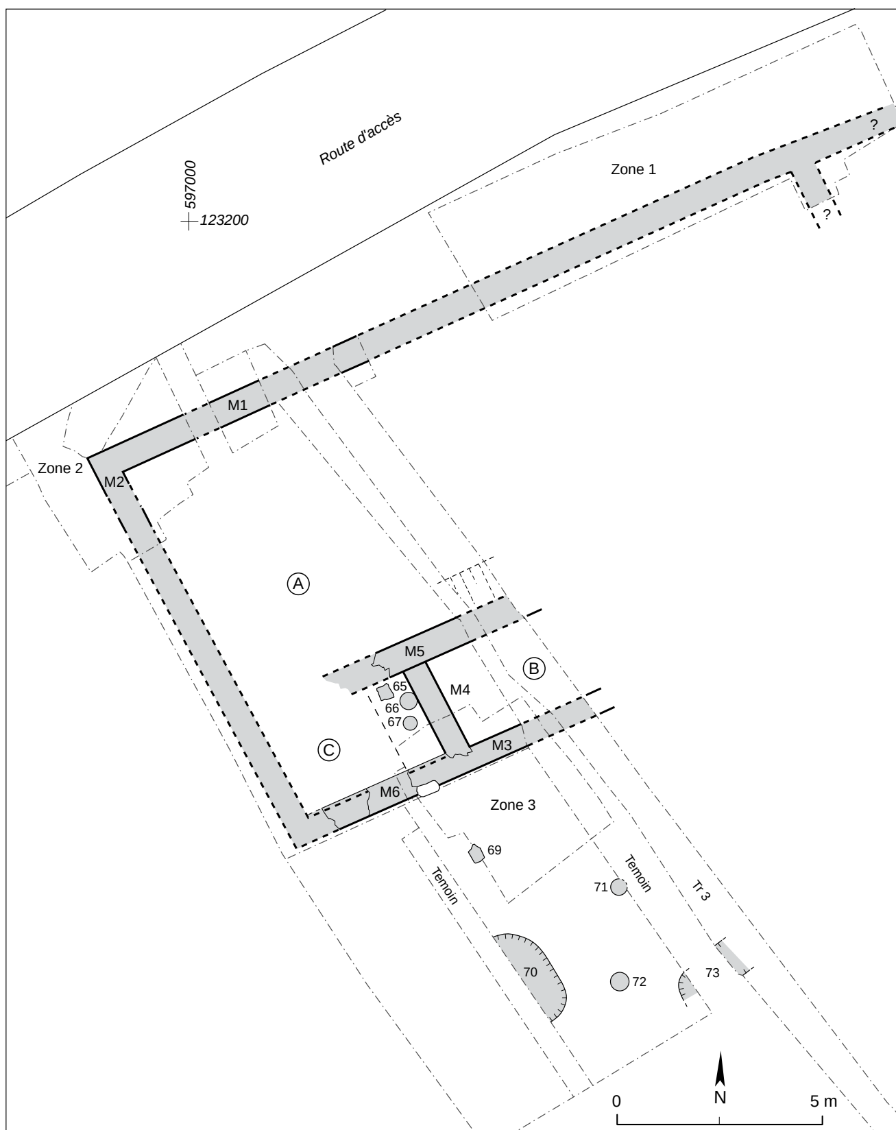
Fig. 16. AF03, maison Aymon. Plan du bâtiment romain.
